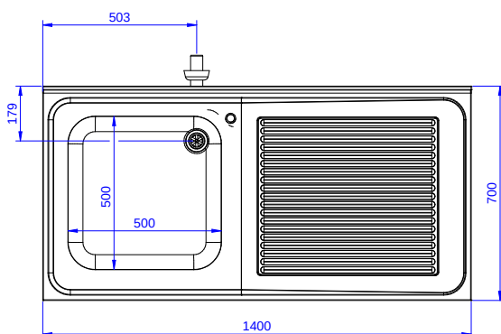
Boven aanzicht
